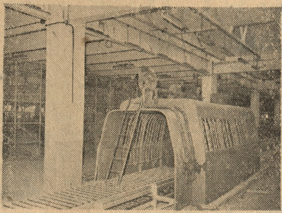
CAF fot. Zygm. Wdowiński Na terenie budowy potężnej Fabryki Samochodów Osobowych na Żeraniu wrą gorączkowe prace montażowe w niedawno wykończonych nowoczesnych halach fabrycznych. Na zdjęciu: spawacz Zdzisław Jagiełło przy montażu kabiny deszczowej, służącej do badania szczelności wozów
