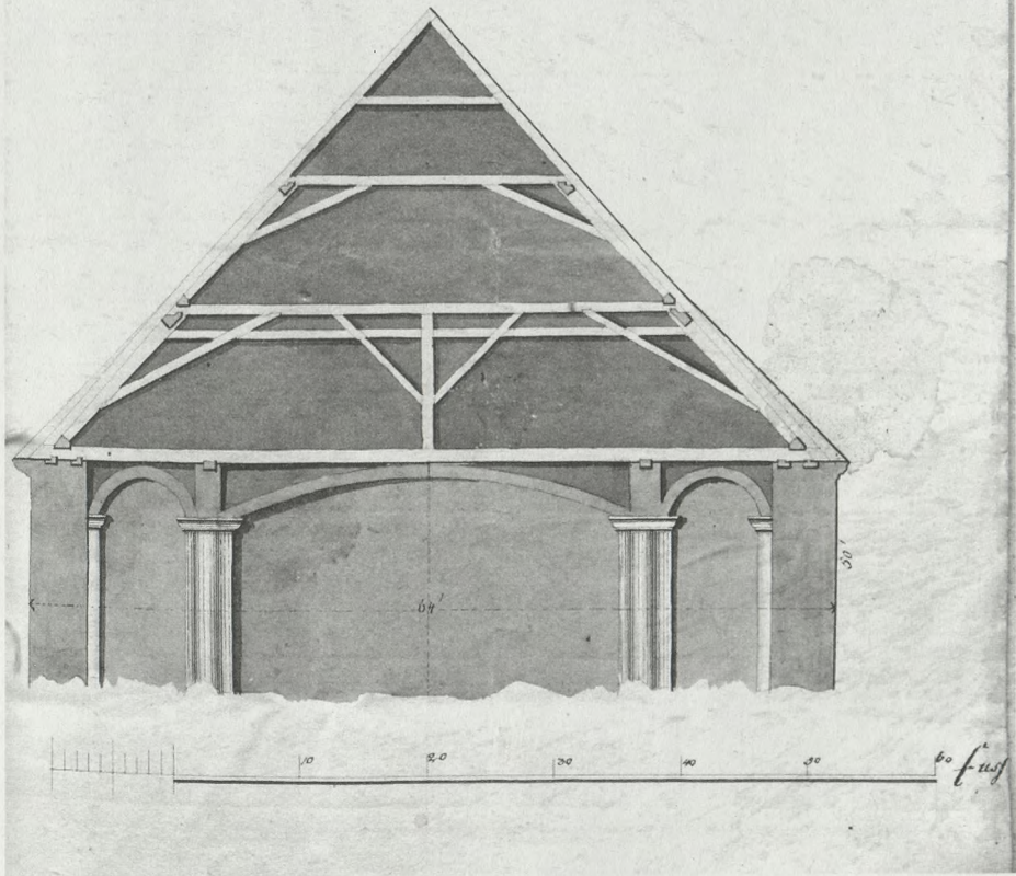
4. Przekrój dachu i sklepień kościoła w Kórniku z 1804 r., „Profil Eines Hauptbinders des Kirchen Daches”,
